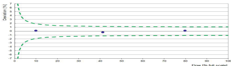
Dokładność przykładowego przepływomierza Flomax w trzech punktach kalibracji - nie więcej niż ±1% wartości mierzonej
