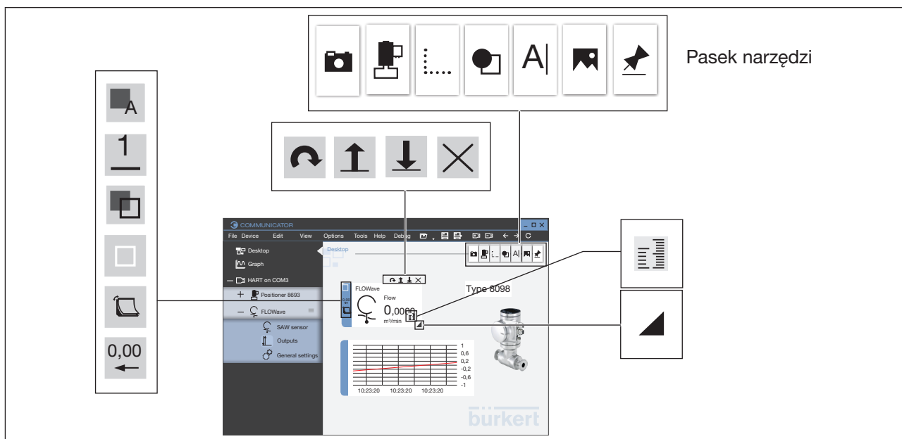
Ilustracja 5: Pasek narzędzi
