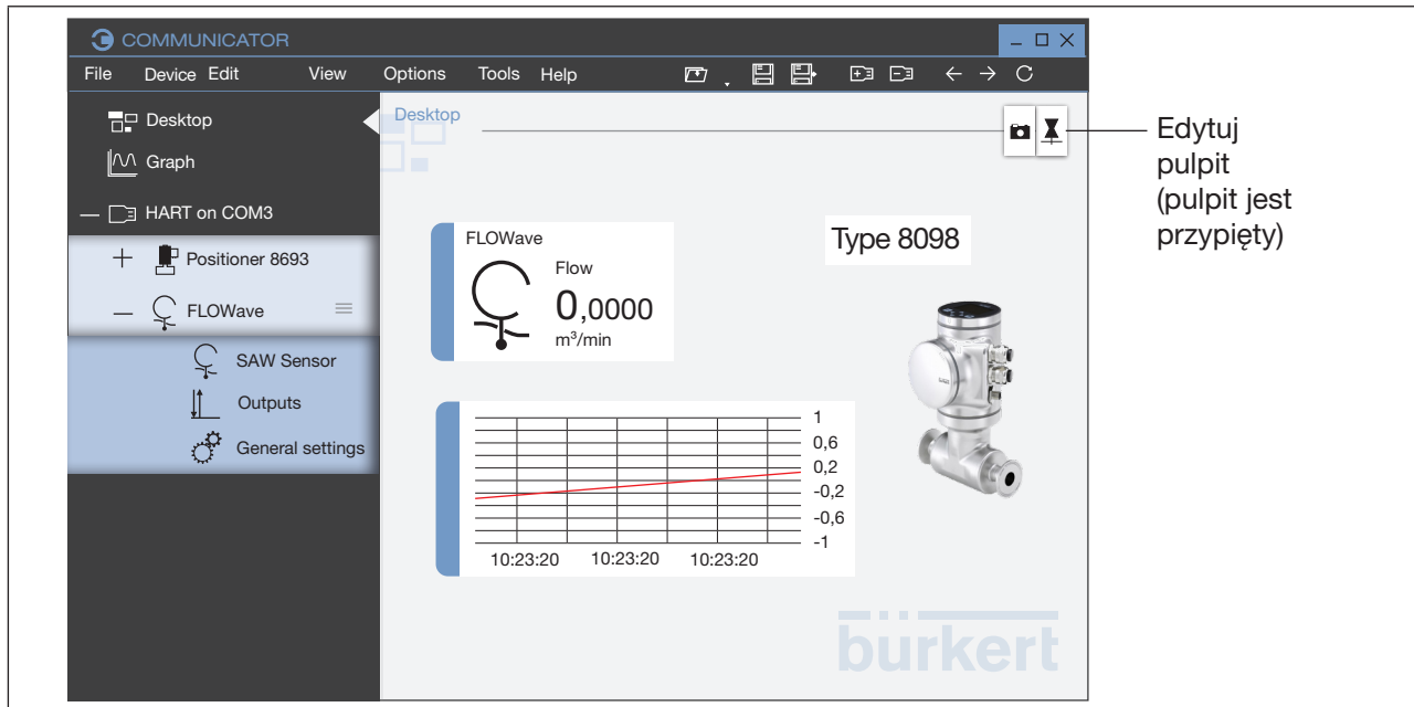
Ilustracja 4: Pulpit (przykład)
