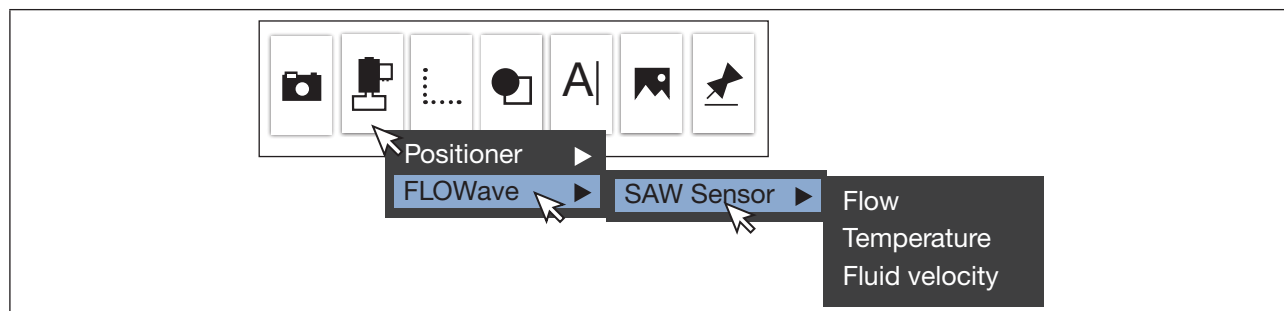
Ilustracja 25: Wstawianie widżetów
