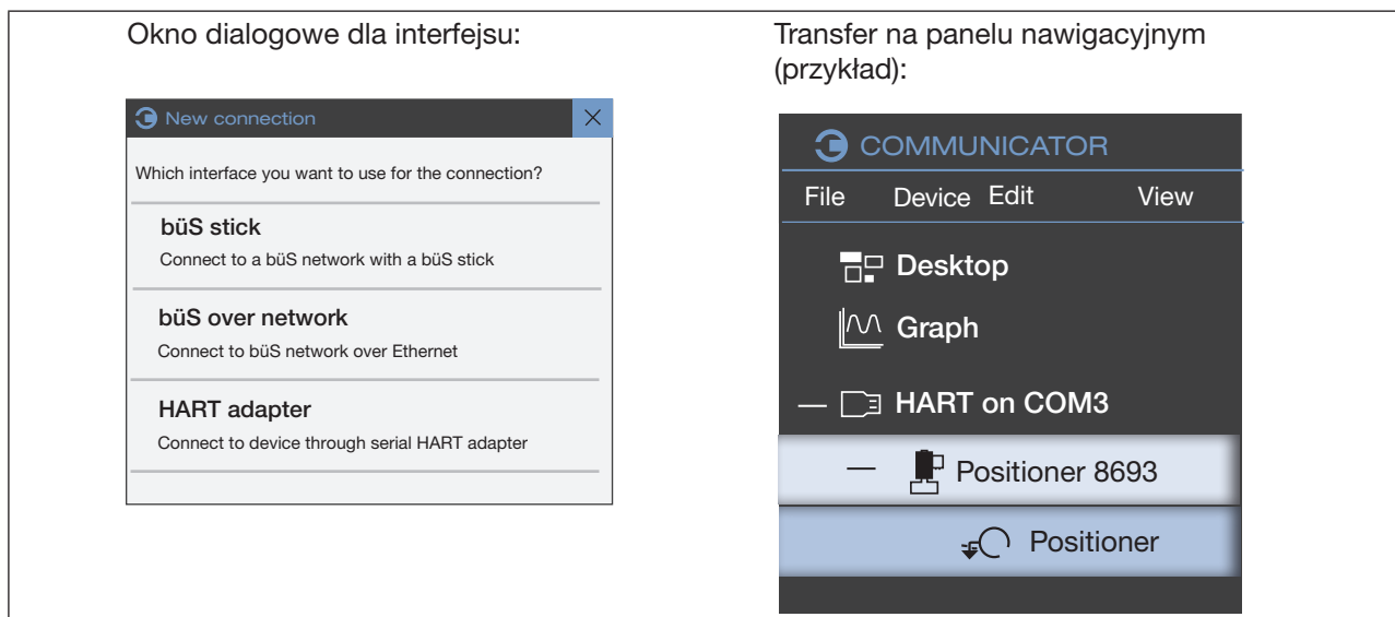
Ilustracja 12: Dodawanie interfejsu
